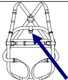
Figura.1.- Arnés con punto de enganche pectoral
